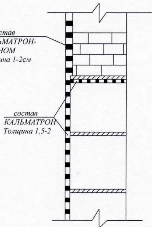
4. Нанесение гидроизоляционного слоя
